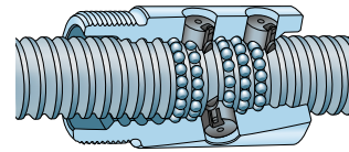
Kugelrückführung
