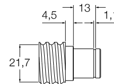
Endenbearbeitung Typ 4A für PND 25 x 5
