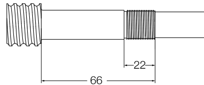
Endenbearbeitung Typ 4A für PND 25 x 5
