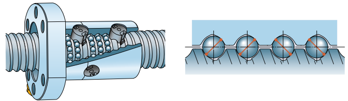
Kugelrückführung
